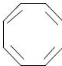
Циклооктатетраен-1,3,5,7
