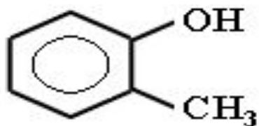
орто-Крезол (1-гидрокси- 2-метилбензол)
