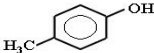
пара-Крезол (1-гидрокси- 4-метилбензол)
