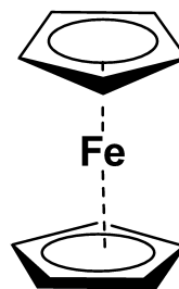
\text{Fe}(\text{Cp})_2 = \text{Ферроцен}
