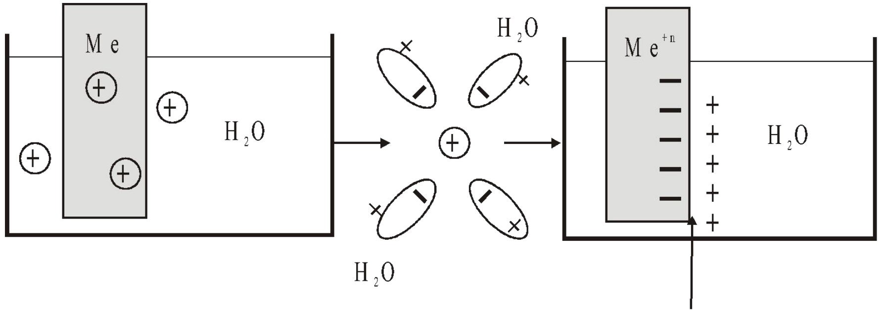
Двойной электрический слой
