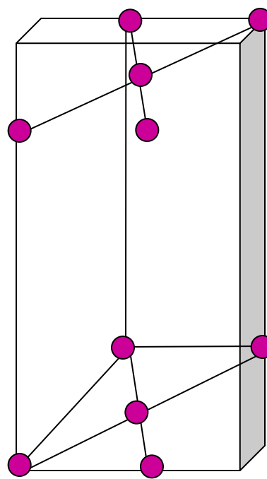
9. Базоцентрированная
