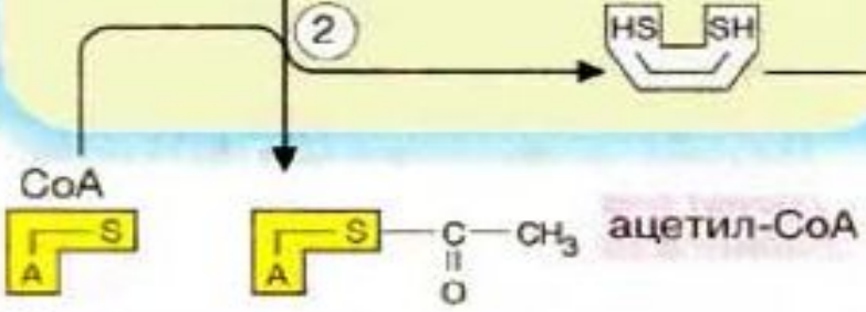
Пируватдегидрогеназа
