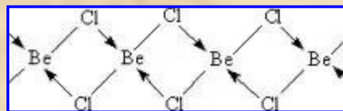
Цепочечная структура хлорида \text{BeCl}_2
