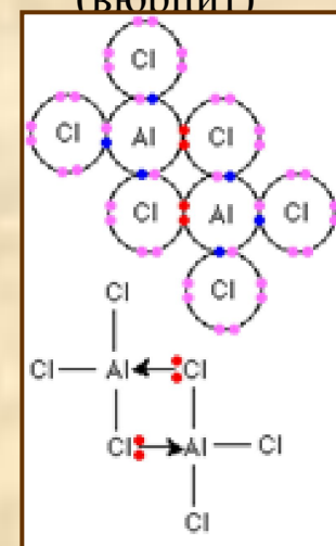
Молекулярная стр-ра \text{AlCl}_3
