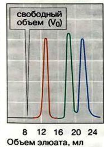
2. График элюирования
