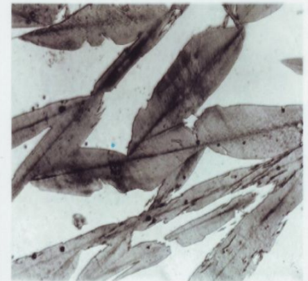
Пластинчатый (двойникованный) мартенсит
