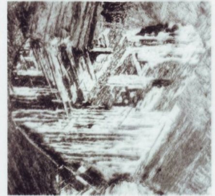
Пакетный (реечный) мартенсит
