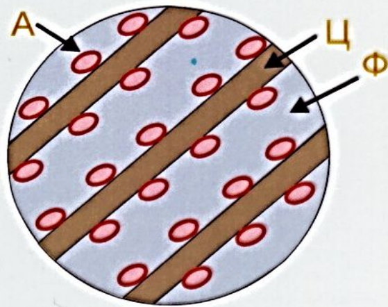
1- Образование зародышей аустенита
