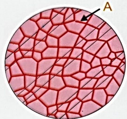
3 - растворение цементита, аустенит неоднороден
