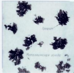
Нетравленый шлиф
