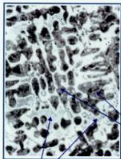
Дозвтектический белый чугун
