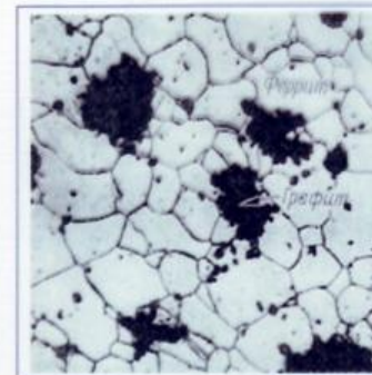
Ковкий ферритный
