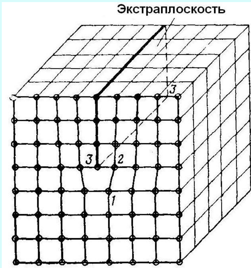
Рис. 4. Дислокации
