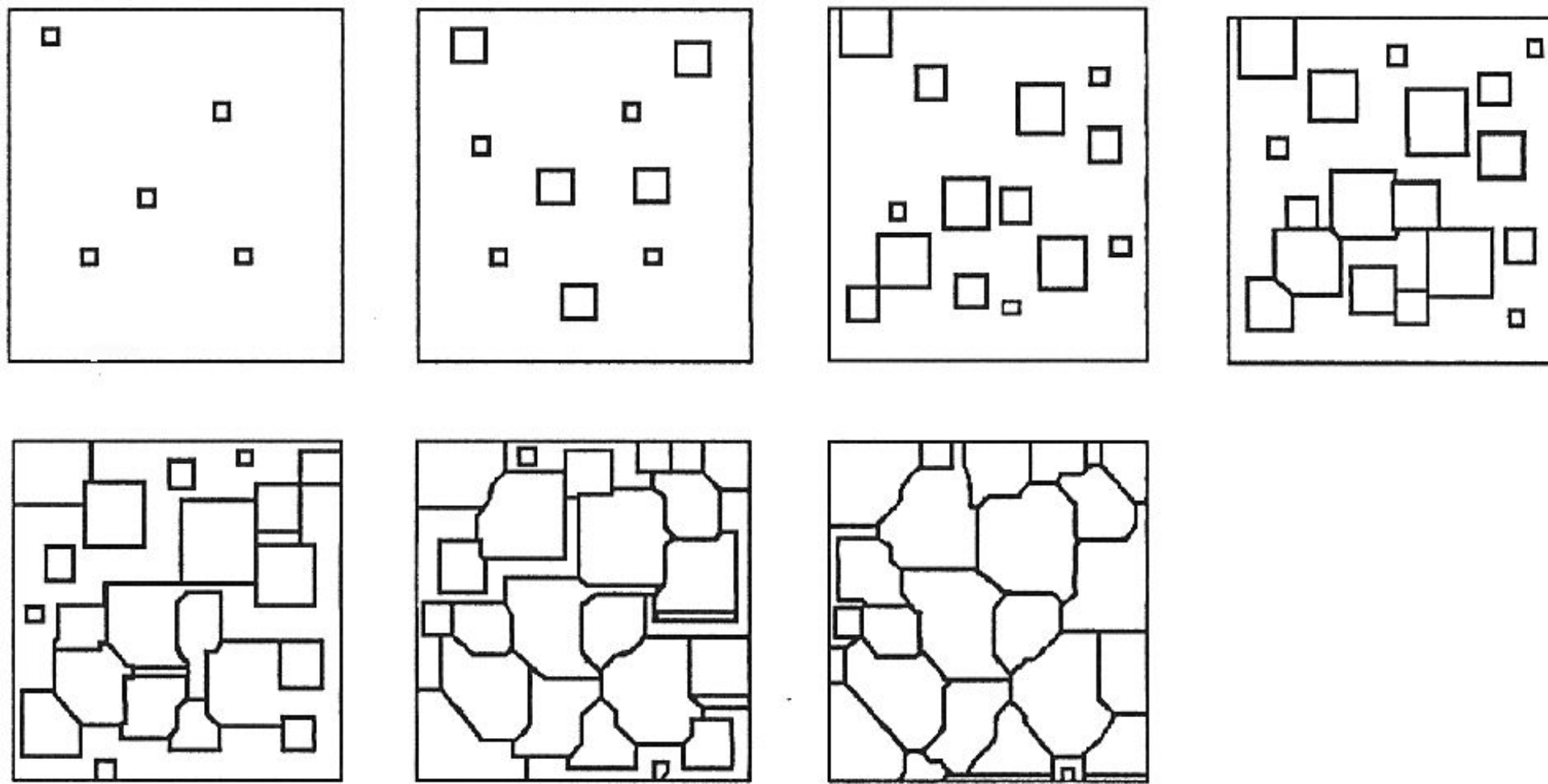
Рис. 6. Схема последовательных стадий процесса кристаллизации сплавов
