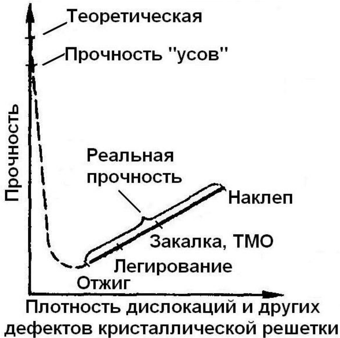
Рис. 5. Схема зависимости прочности сплавов от количества дефектов
