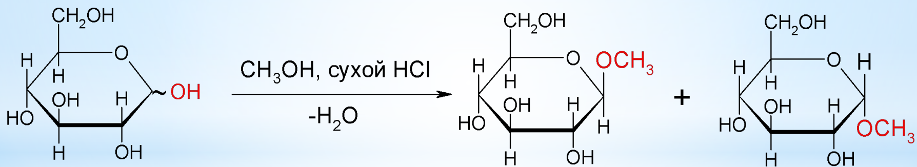
D-глюкопираноза
