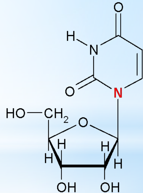
уридин
