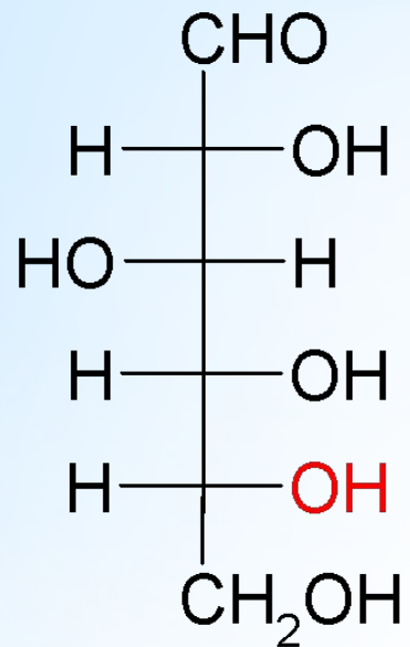
D -глюкоза
