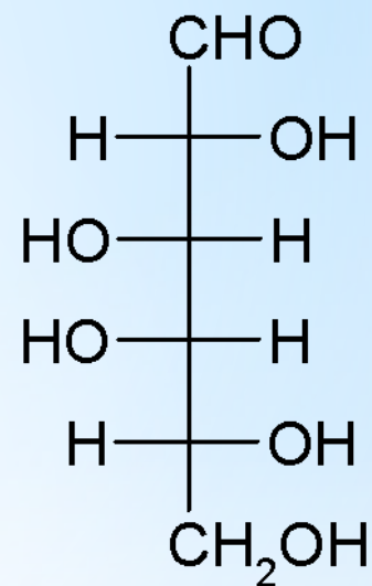
D-галактоза
