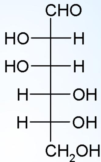
D-манноза
