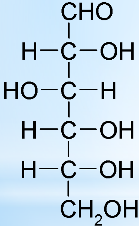
глюкоза
