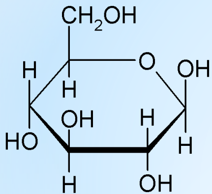
β-D-глюкопираноза
