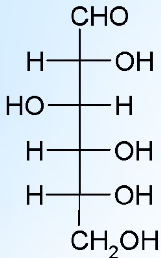
D-глюкоза
