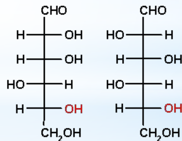
D-гулоза D-идоза
