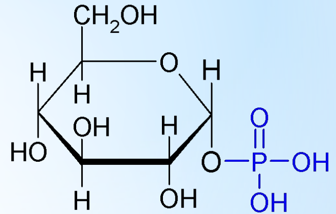
D-глюкозо-1-фосфат
