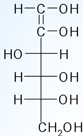
ендиольная форма
