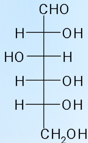
глюкоза
