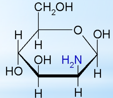
D -маннозамин
