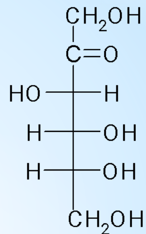
фруктоза
