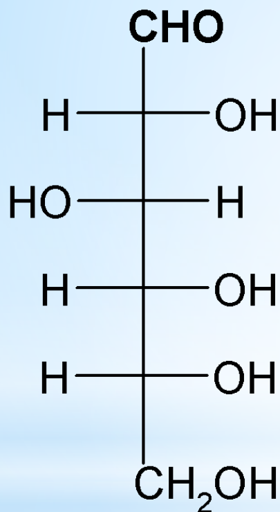
глюкоза
