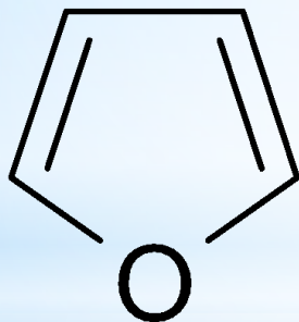
фуран
