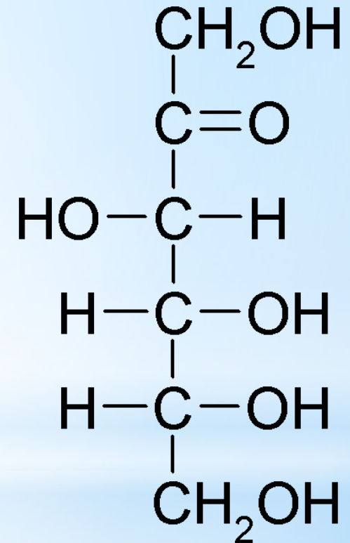
фруктоза
