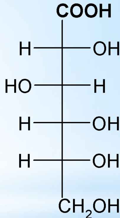
глюконовая кислота
