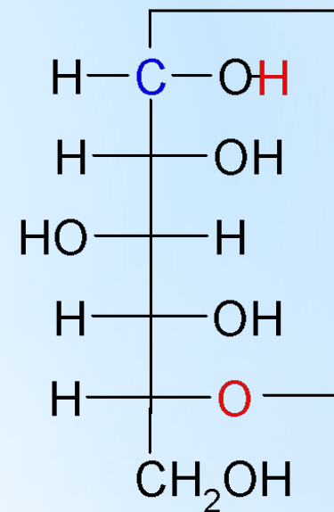
\alpha -аномер
