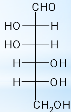
манноза
