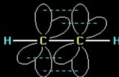
Атомно-орбитальная модель
