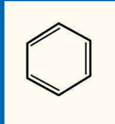
Схематическое изображение бензольного кольца
