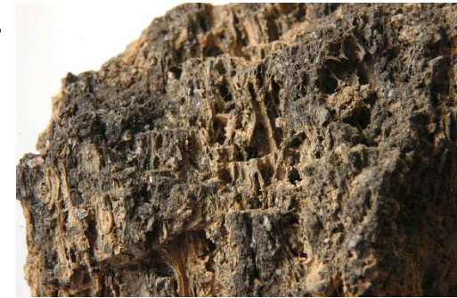
Базальты
