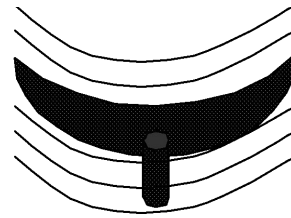
лополит
