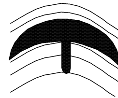
лакколлит
