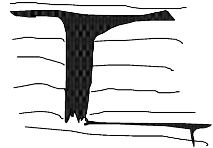
диатрема и подводящий силл
