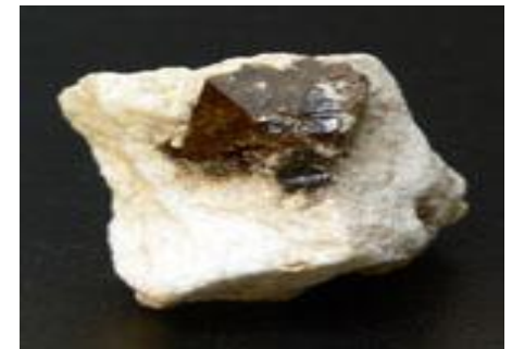
Циркон \text{Zr}[\text{SiO}_4]
