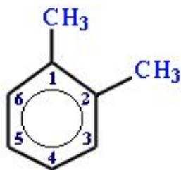
1,2-диметилбензол
