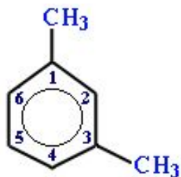
1,3-диметилбензол
