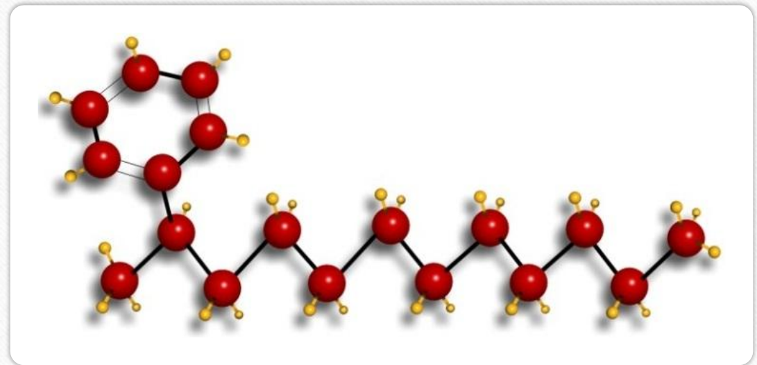
Алкилбензолы
