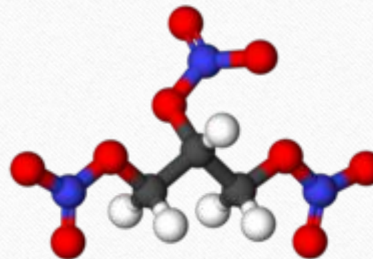
Нитроглицерин
