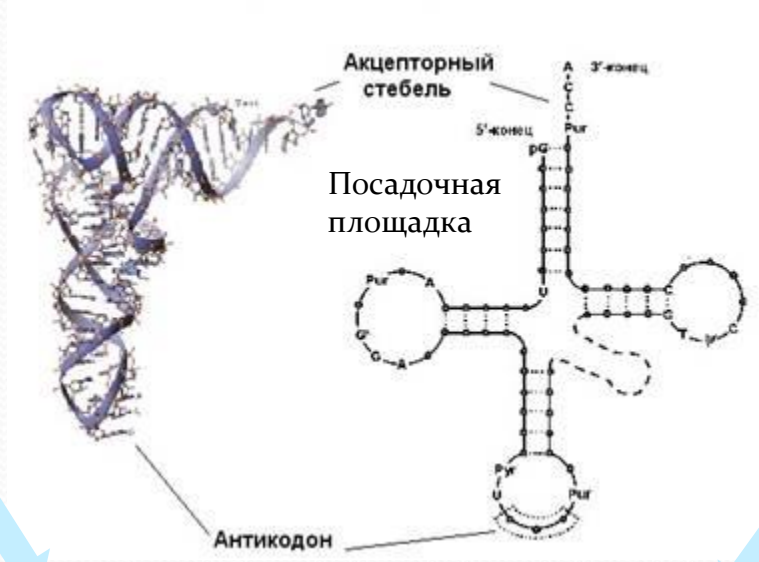
СТРУКТУРА тРНК
