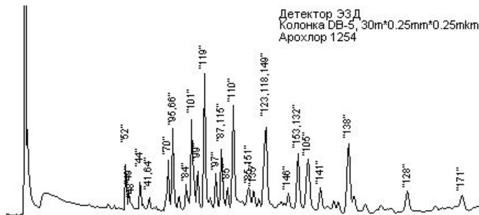
Хроматограмма
