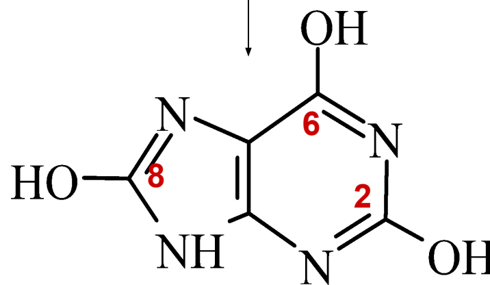
Енольна форма
