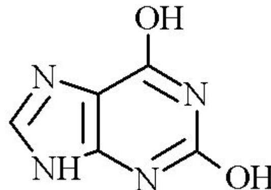
Ксантин
