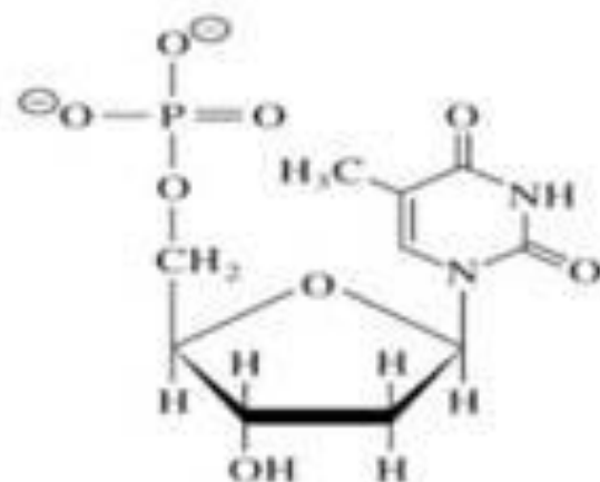
дТМФ
