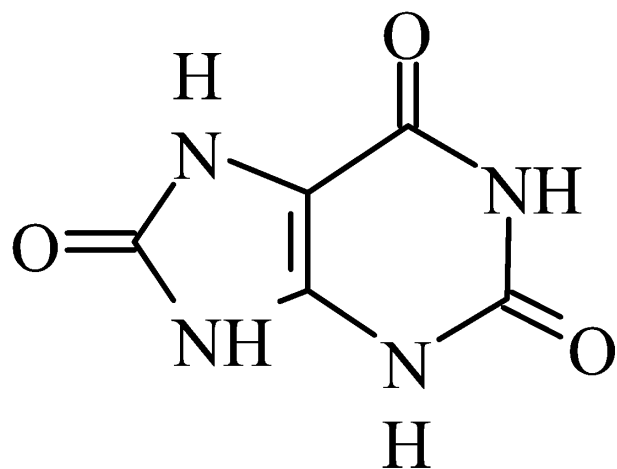
Кето форма
