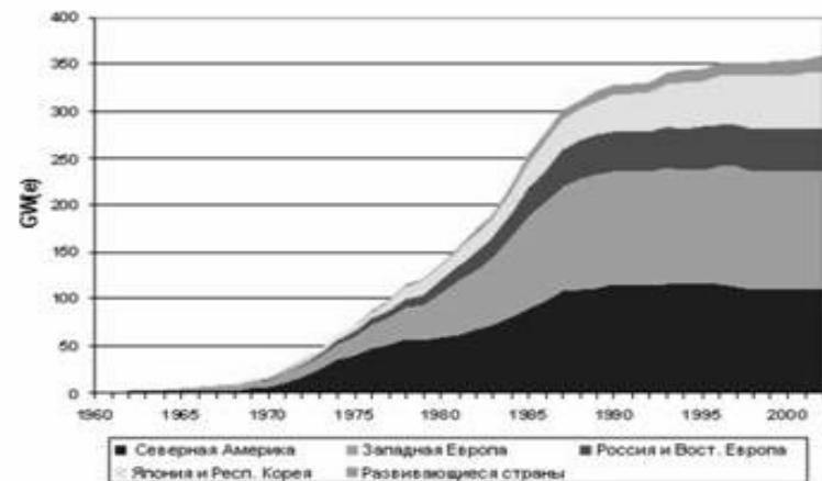
Энергетическая мощность действующих атомных электростанций в мире
