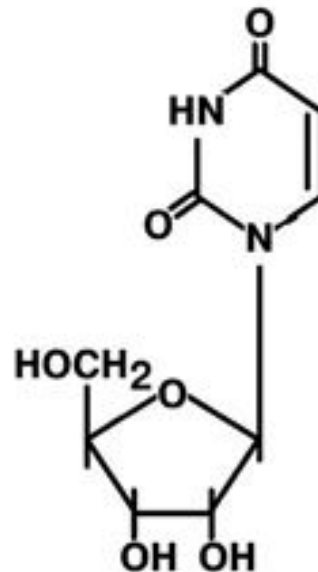
Уридин
