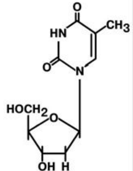
Тимидин
