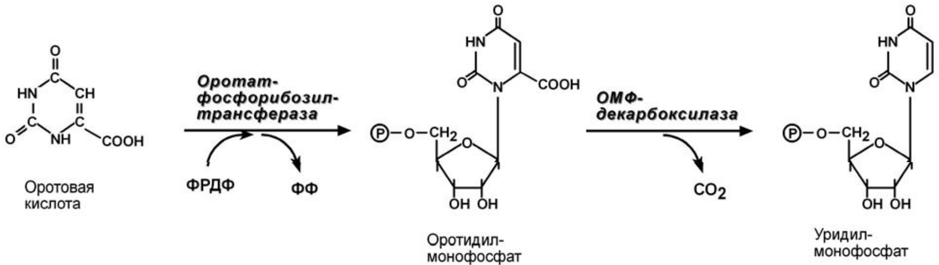
Синтез уридилмонофосфата
