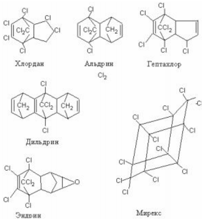
Рис. 1. Пестициды – стойкие органические загрязнители.
