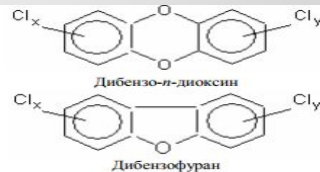
Рис. Химическая структура полигалогенированных дибензо- para -диоксинов и дибензофуранов.
