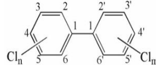
Рис. 1. Структура молекул полихлорированных бифенилов.
