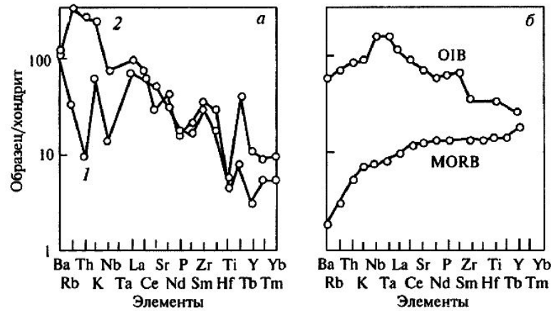
Рис. 1.7. Спайдер-диаграммы, нормированные по хондриту (значения для нормализации по Thompson, 1982) для средних составов нижней 1 и верхней 2 континентальной коры (а) и для средних составов базальтов срединно-океанических хребтов и океанических островов (б) [220]
