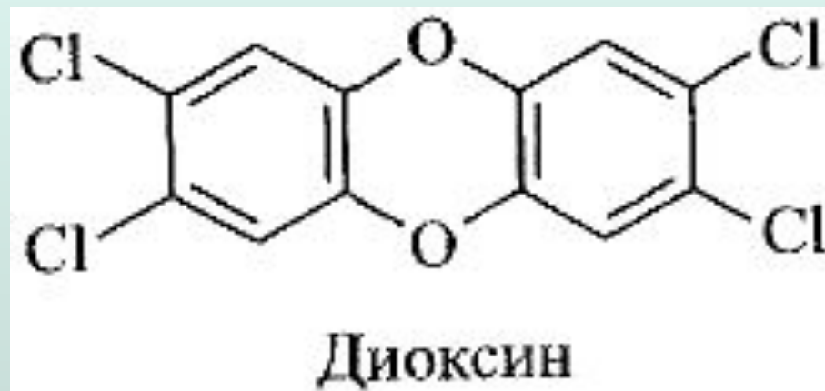
Диоксин 2,3,7,8-тетрахлордibenзо-p-диоксин
