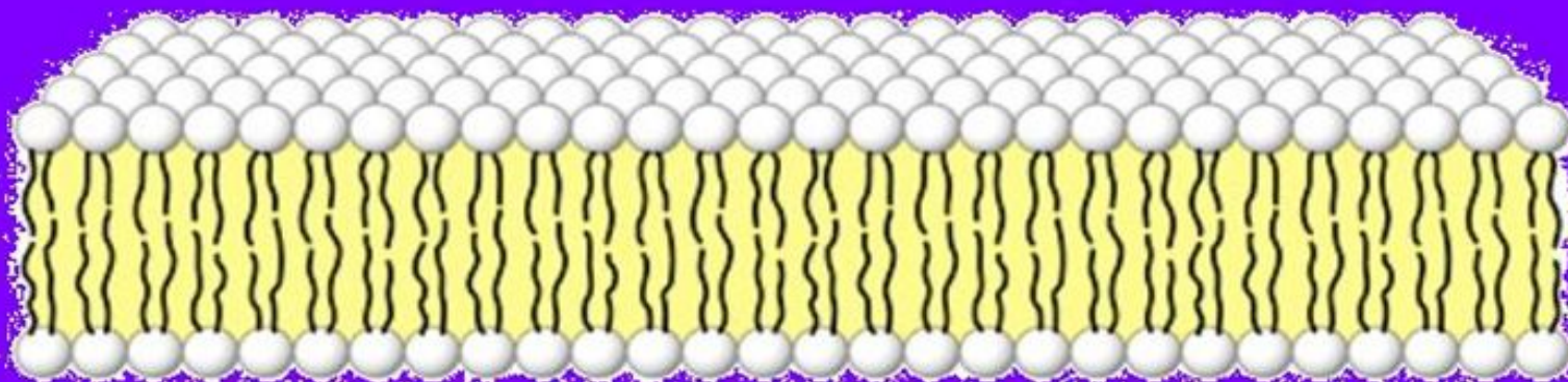
бислой фосфолипида
