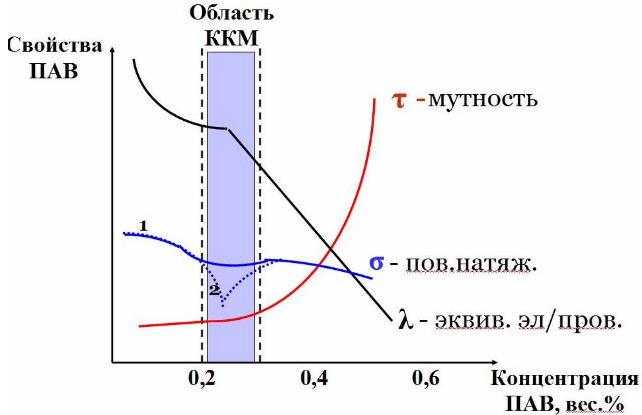
Рис. XII.3 Изменения свойств ПАВ в области ККМ.
