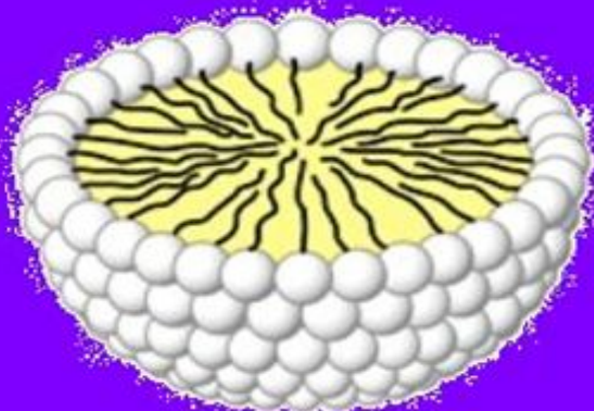
мицелла
