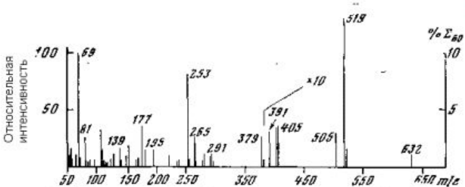
Рис. 2. Масс-спектр пента-О-трифторацетата ксилита (Chizhov O.S. et. al.- Organic Mass Spectrometry, 1969, vol. 2, p. 947)
