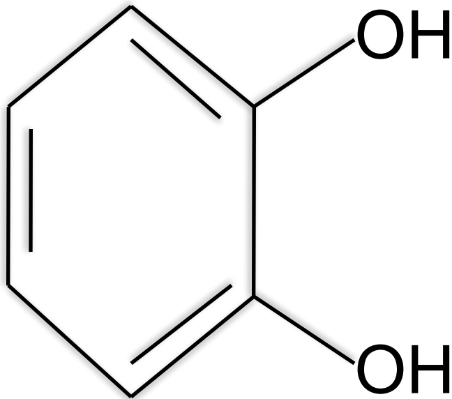
Пирокатехин
