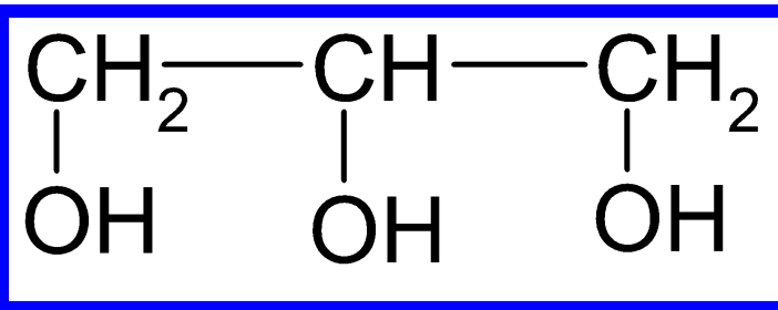
Пропантриол-1,2,3
