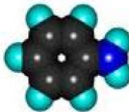
модель молекулы
