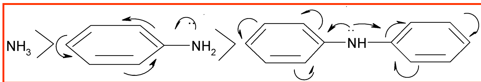
фениламин
