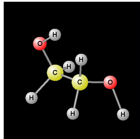
Этандиол-1,2
