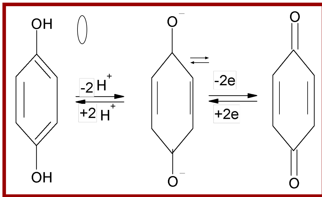
ХИНОН
