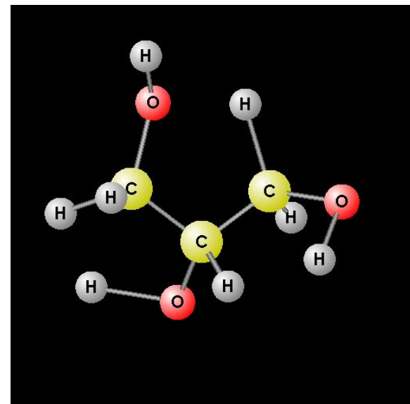
Пропантриол-1,2,3
