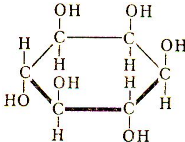
Мезоинозит.
