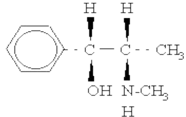
Эфедрин
