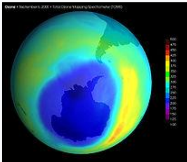
Изображение антарктической озоновой дыры, сентябрь 2000.
