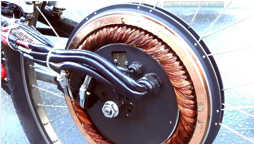
Мотор-колесо Дуюнова 12кВт
