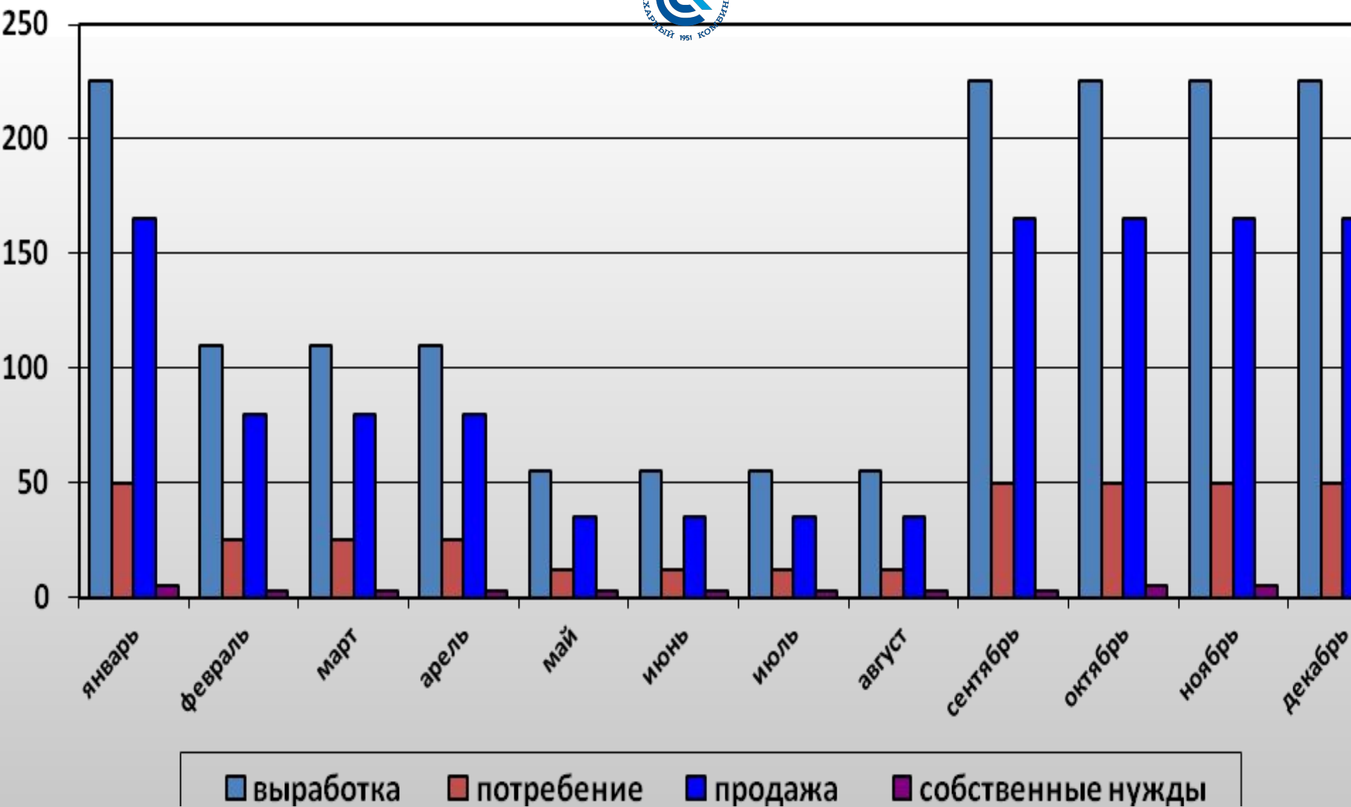
Баланс электрической энергии в рассматриваемом варианте реконструкции
