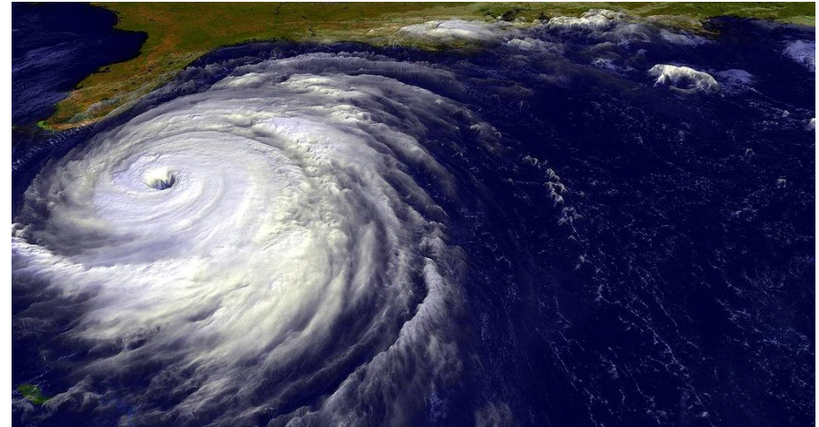
Тайфун
