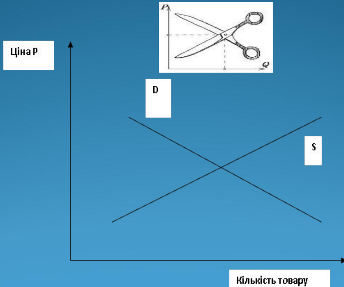
Рис. 3 “Хрест” Маршалла
