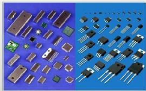
Полупроводники
