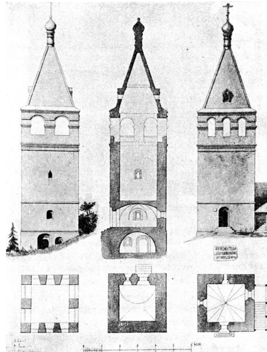
Обмеры колокольни Дудина монастыря 1876 г.; Источник: Известия ИАК от 1 января 1912 г.
