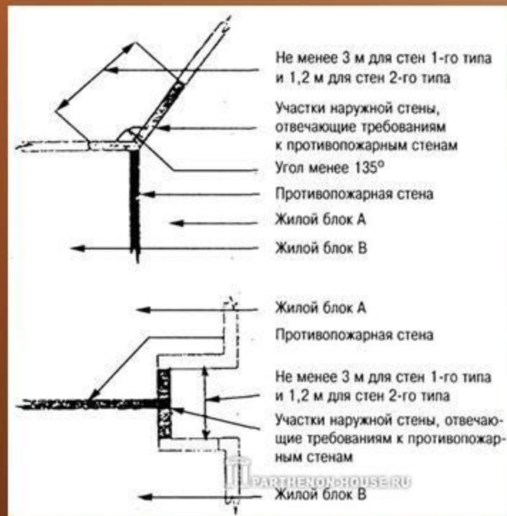
Варианты устройства противопожарной стены
