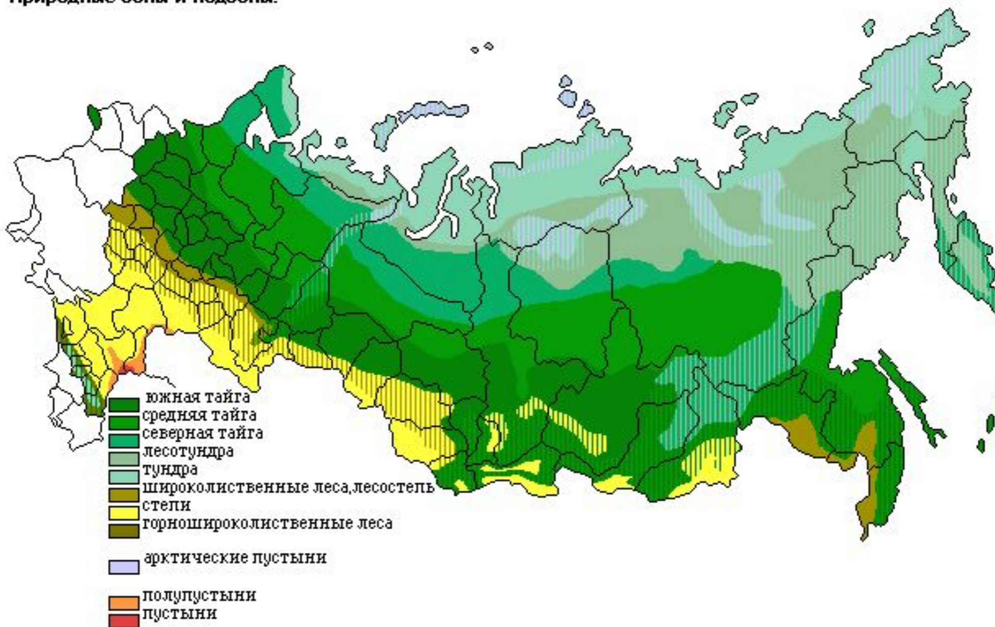
Природные зоны и подзоны.
