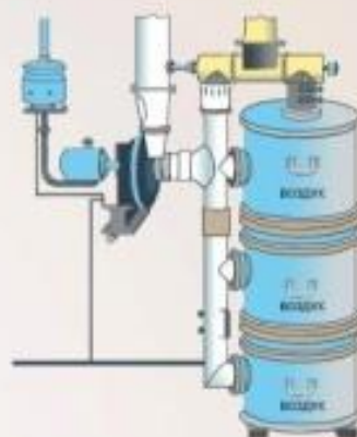
ФИЛЬТРОВЕНТИЛЯЦИОННЫЙ АГРЕГАТ
