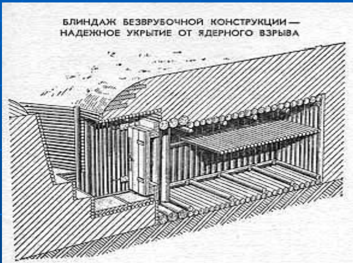
Блиндаж
