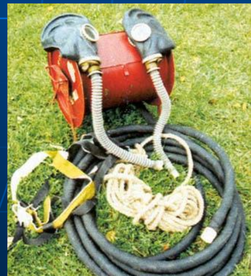
Противогазы шланговые ПШ-1Б и ПШ-РВ
