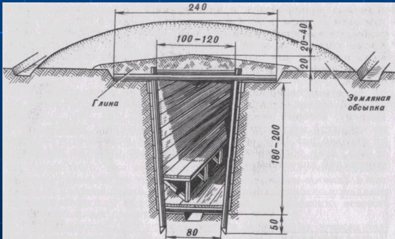
Перекрытая щель
