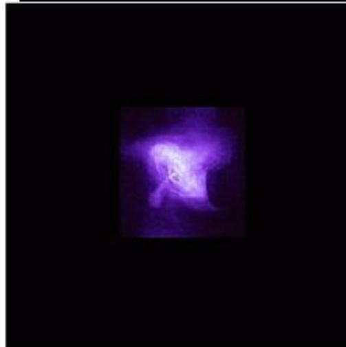
Мягкое рентгеновское
