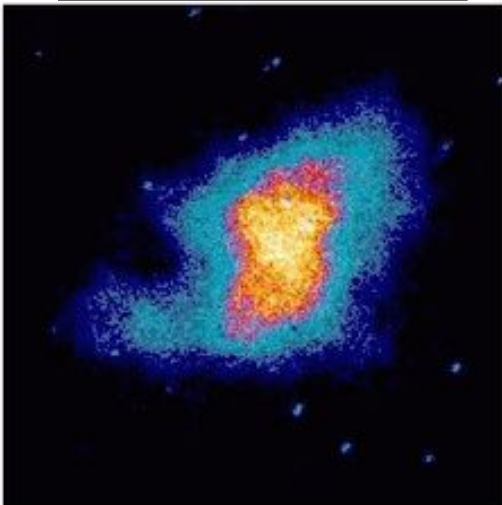
Ультрафиолет
