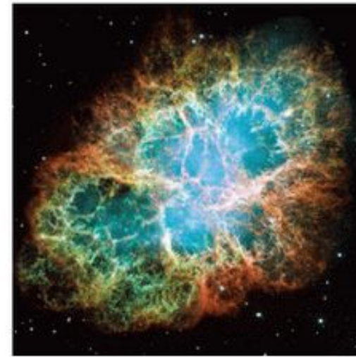
Видимый свет
