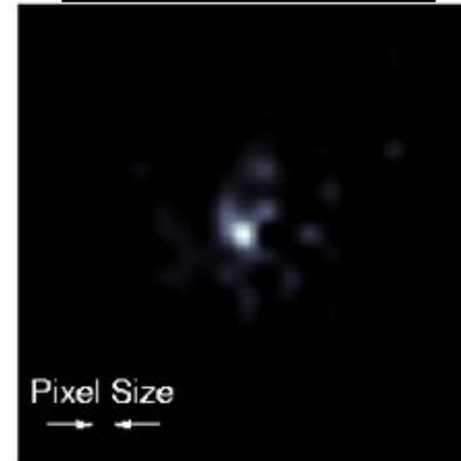
Жёсткое рентгеновское
