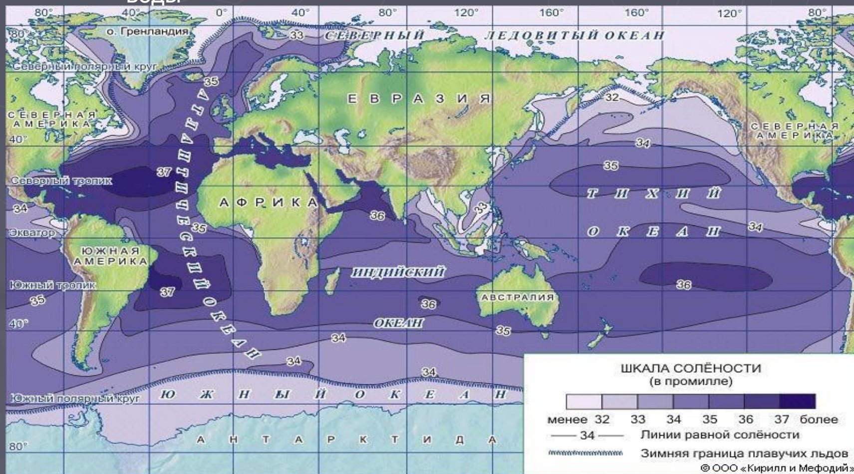
Карта солёности вод Мирового океана в промилле (количество грамм соли на килограмм воды).
