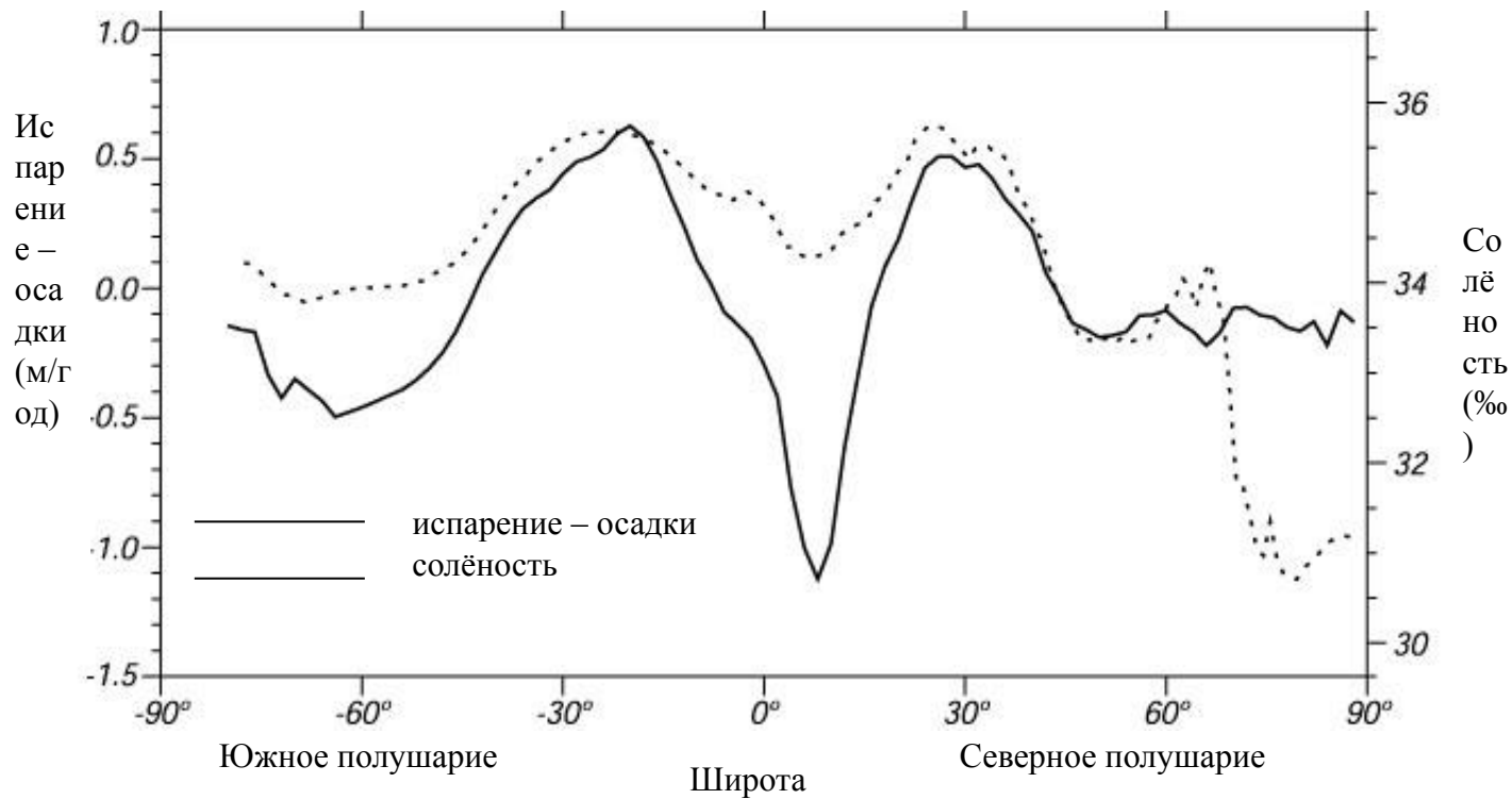
Рис. 4.1. Широтное распределение солёности, и разности между испарением и осадками.
