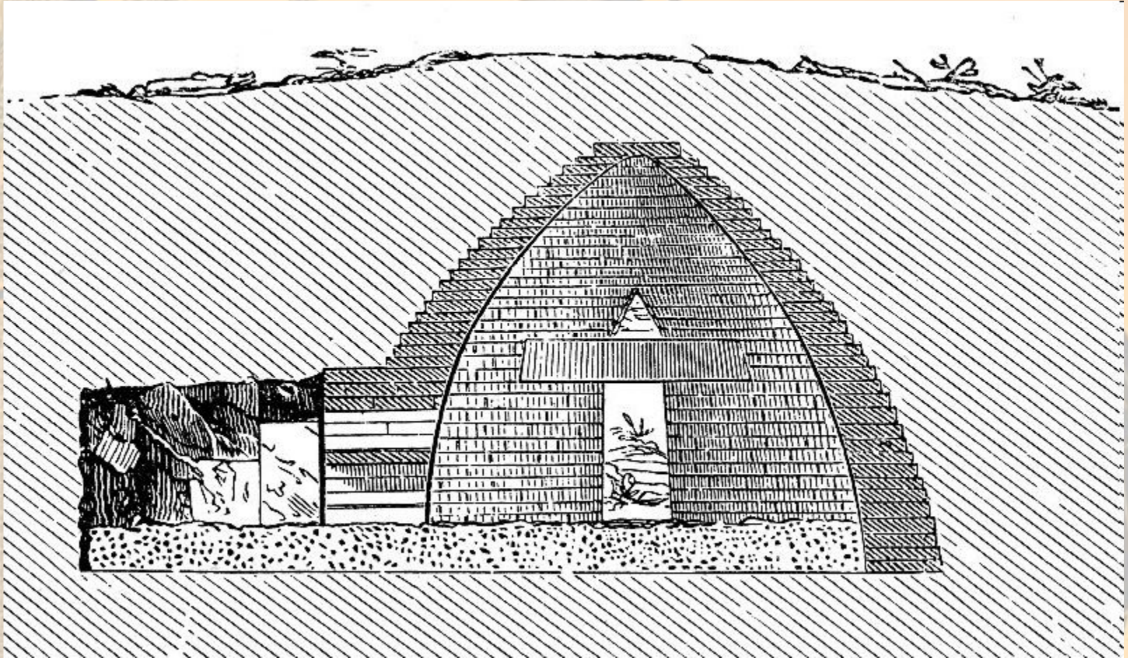
Гробница Атрея в разрезе
