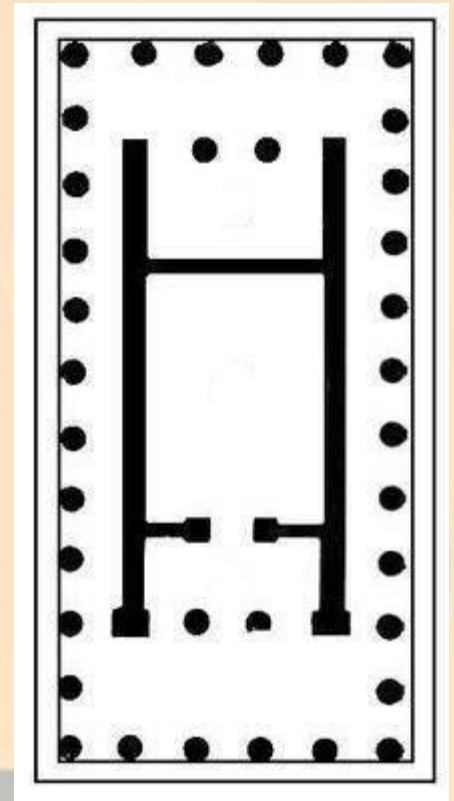
Периптер План
