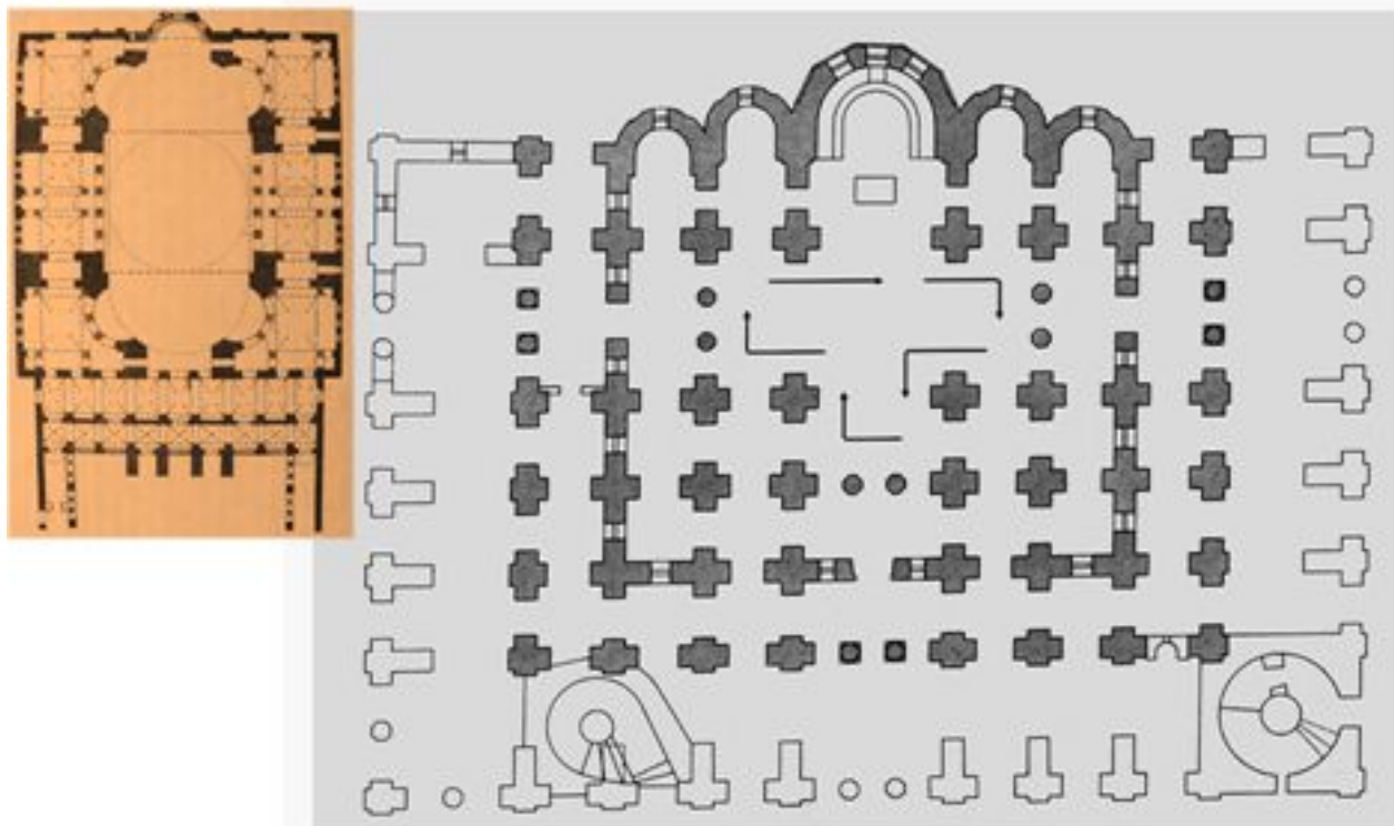
Софийский собор в Киеве 1017-1037.
