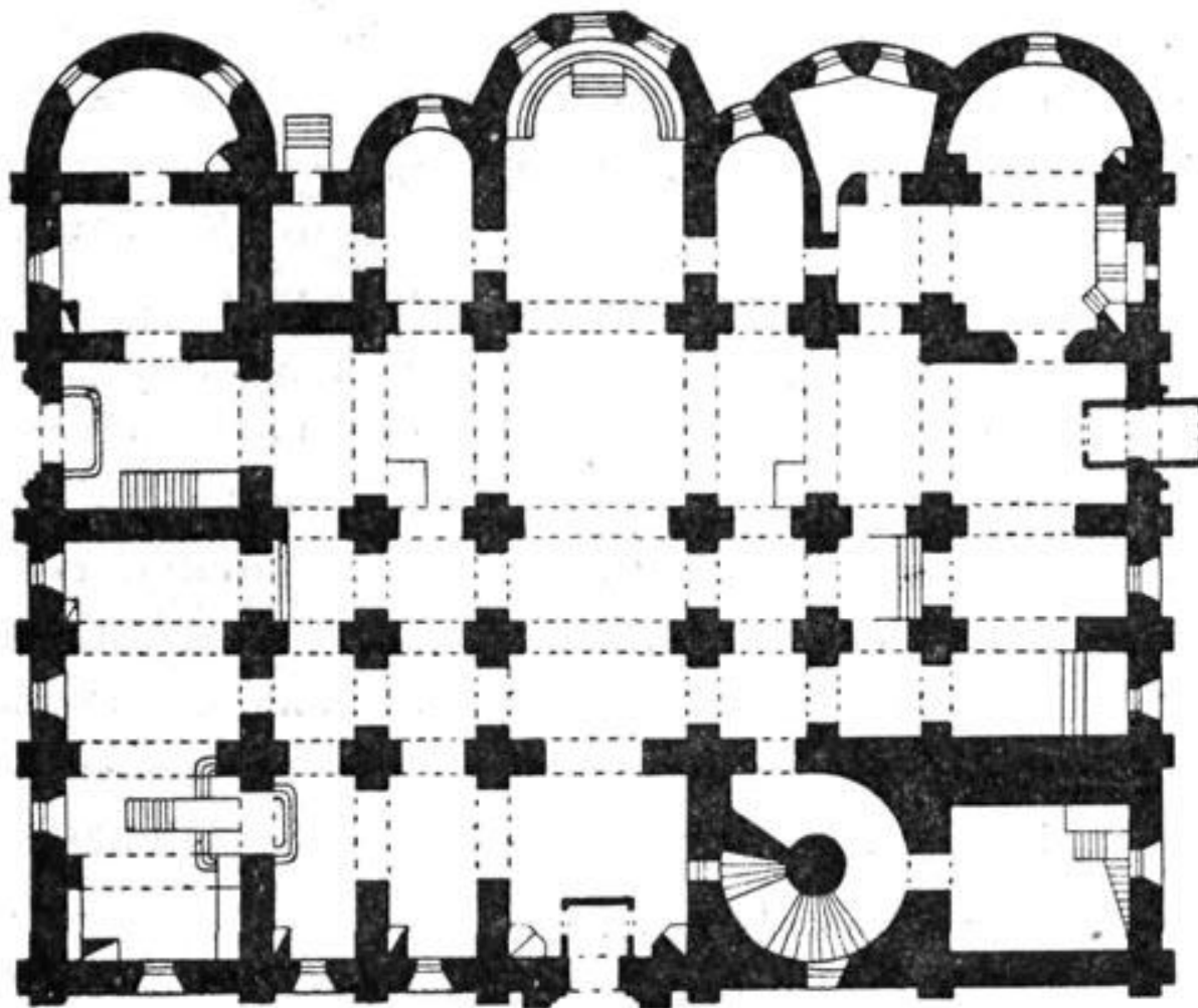
Храм св. Софии в Новгороде. План. 11 в
