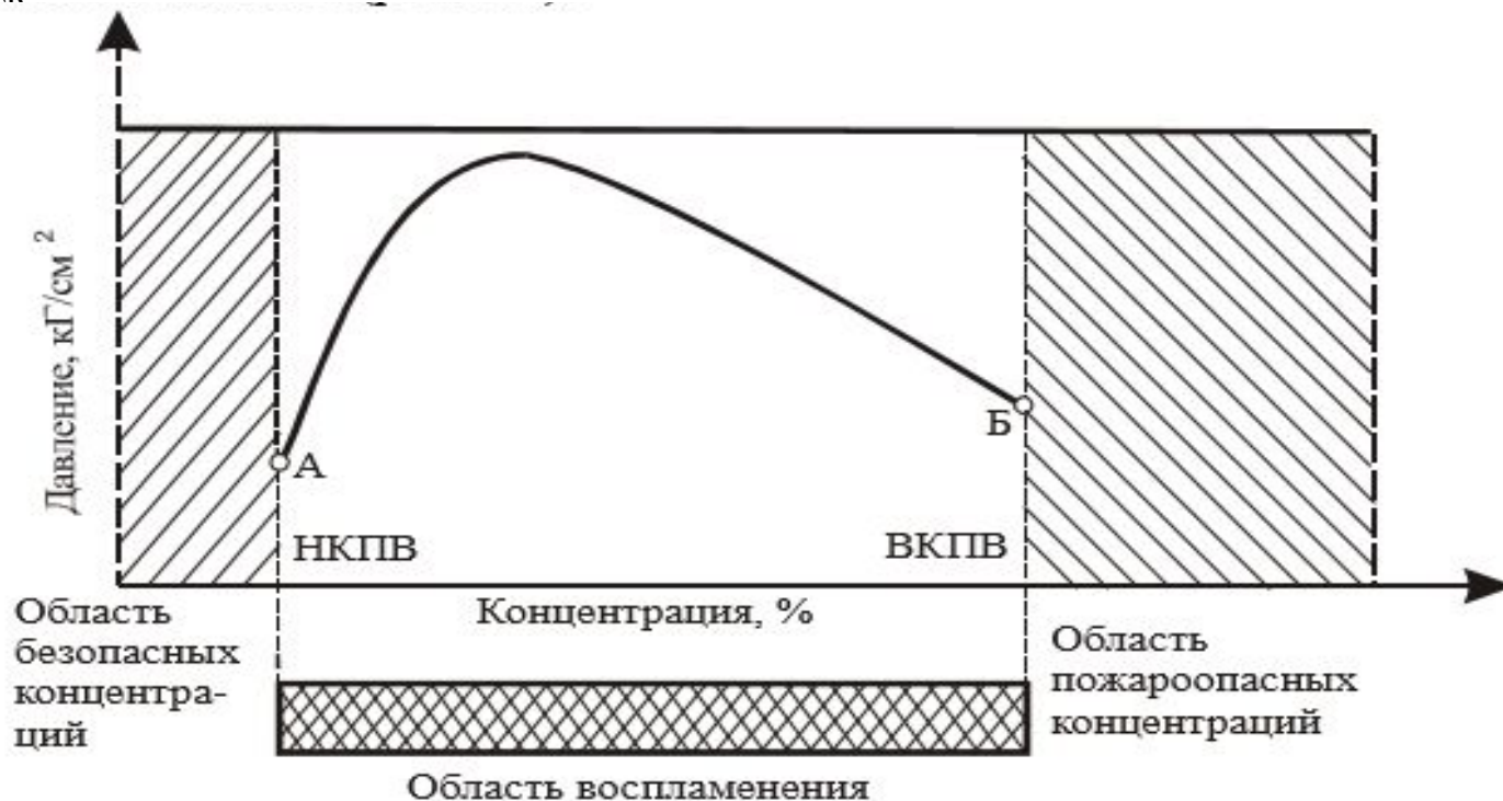
Рис. 2.1. Зависимость давления при взрыве горючих газопаровоздушных смесей от концентрации горючего в смеси
