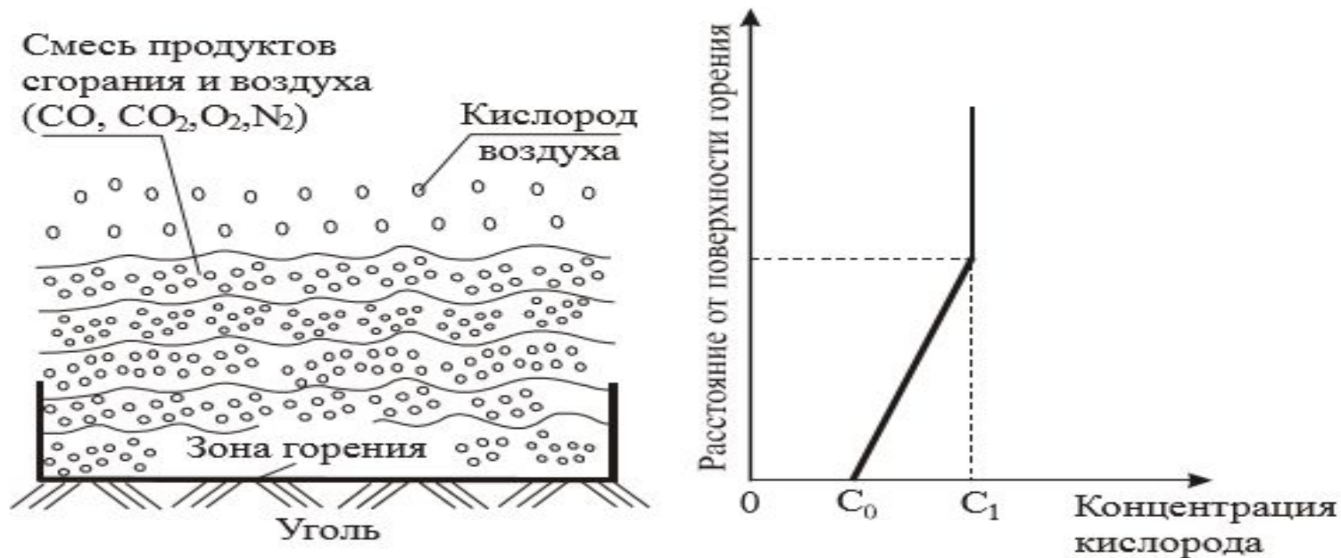
Рис. 1.4. Схема диффузии кислорода в зону горения твердого вещества (гетерогенное горение)
