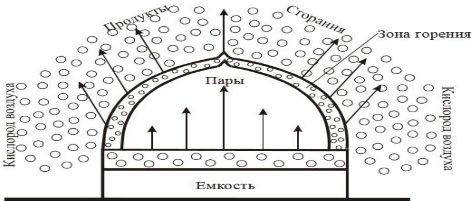
Рис. 1.3. Схема процесса горения паров или газов
