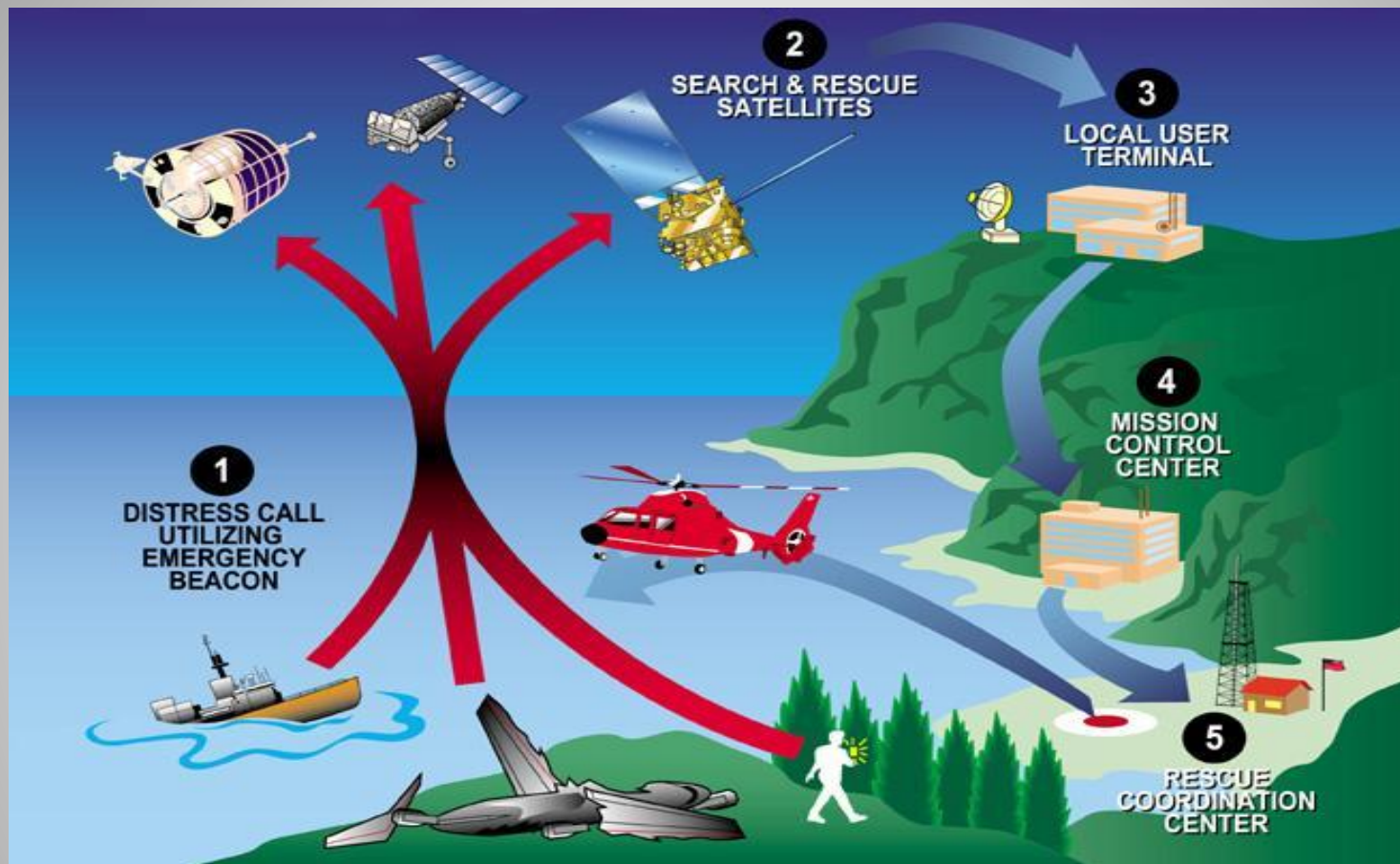
СИСТЕМА «КОСПАС-SARSAT»
