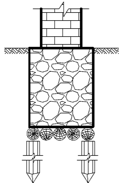
со сваями
