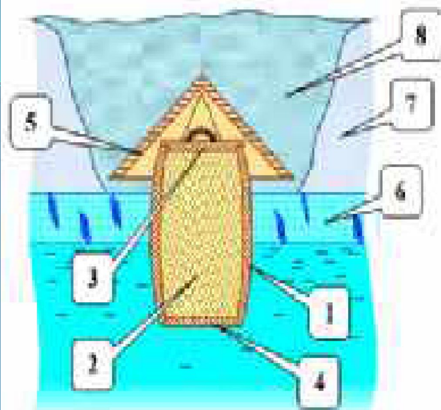
Рис. 5.34 Утепление проруби при вмораживании бочки
