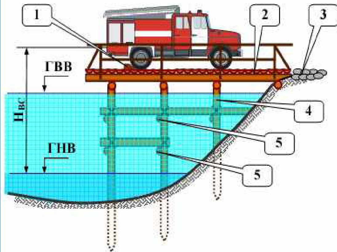
Рис. 5.33 Пожарный пирс
