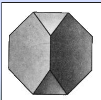
Усеченный тетраэдр
