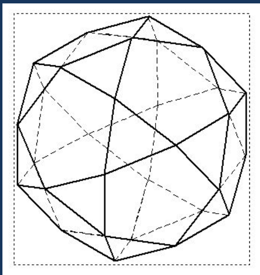
Икосододекаэдр р
