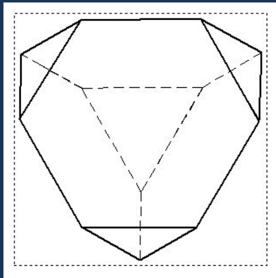
Усеченный тетраэдр
