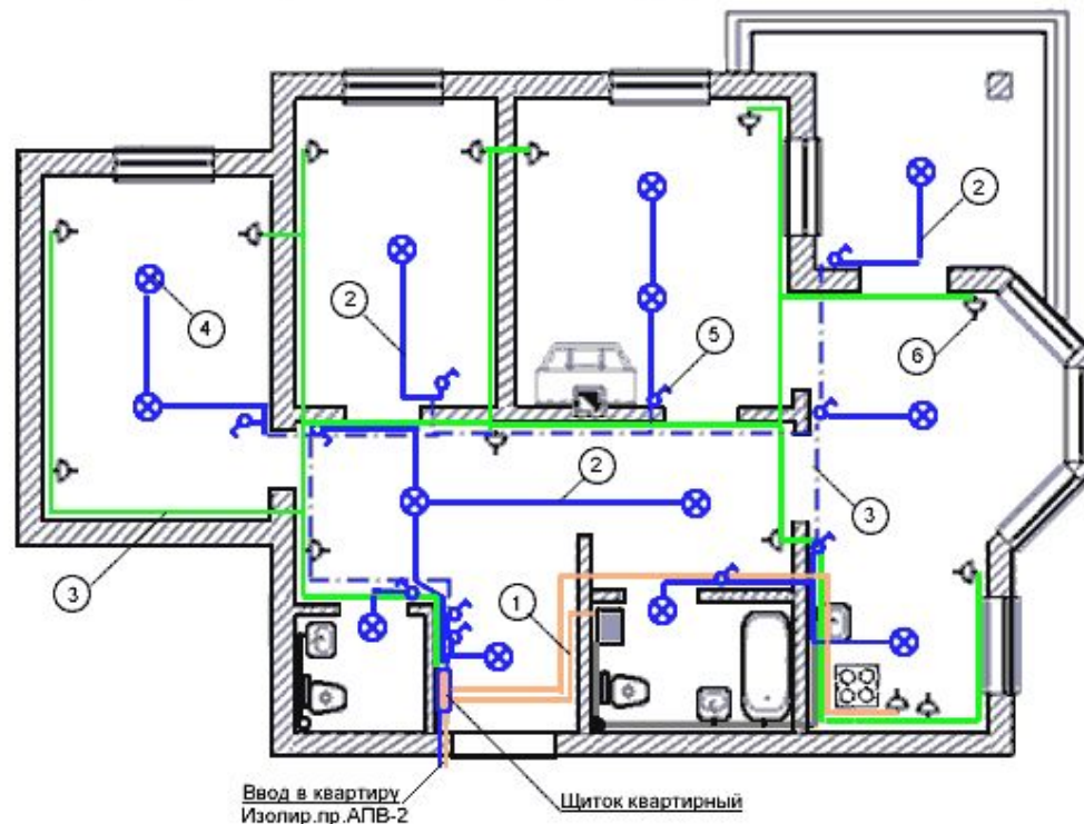
П л а н к в а р т и р ы разводка скрытой электропроводки
