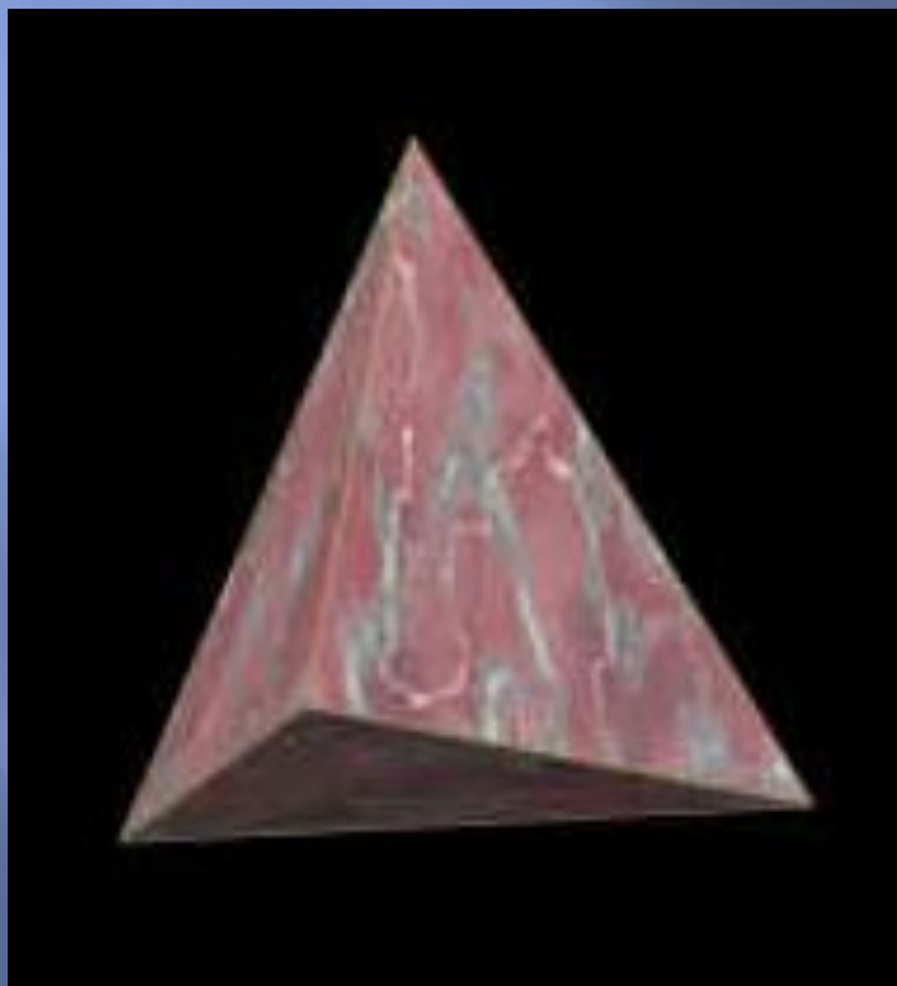
ТЕТРАЭДР
