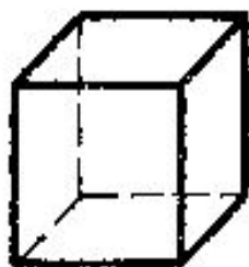
Куб
