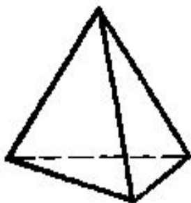
Тетраэдр
