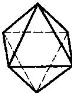
Октаэдр
