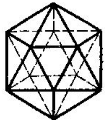
Икосаэдр
